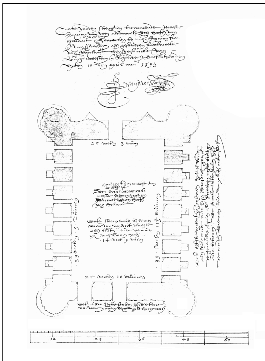
"Caerte van den steenoven toecomende Meester Symon van Veen", Symon Fransz. van Merwen, 10 april 1593. Deze steenoven beschikte aan beide kanten over 8 stookgaten, ook wel vuurmonden genoemd.
