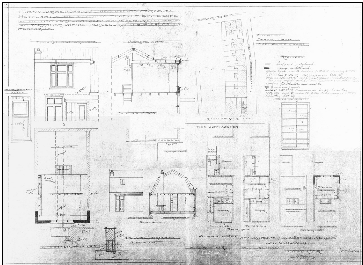
Bouwtekening van Jan Verhagen Jr.: Plan voor het opbouwen van de achtergevel
